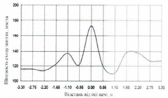
Рис. 6.3. Відеокадр 2 - «Швидкість сходу»
