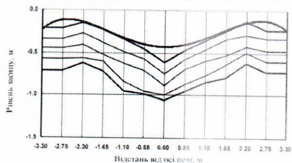
Рис. 6.2. Видеокадр 1 - «Профили засыпи шихты»
