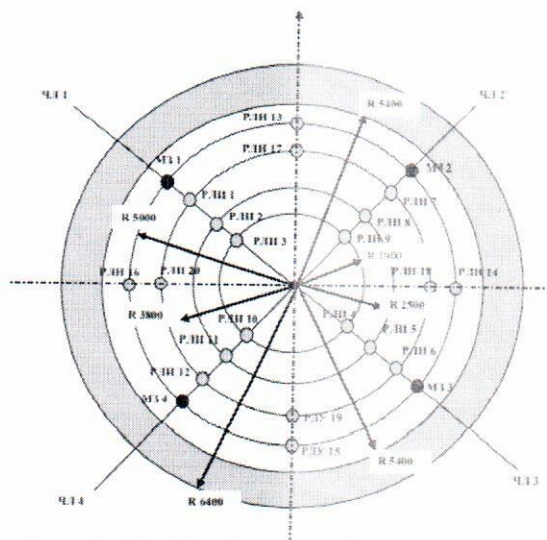
Рис. 6.1. Розміщення радіолокаційних рівнемірів РДУ-X2 на колошнику ДП-9
