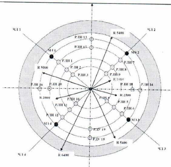
Рис. 5.26. Размещение радиолокационных уровнемеров РДУ-X2 на колошнике ДП-9
