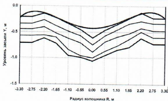
Рис. 5.39. Видеокадр 1 – «Профили засыпи шихты»
