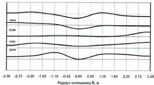
Рис. 5.41. Відеокадр 3 – «Толщини шарів порцій по діаметру»
