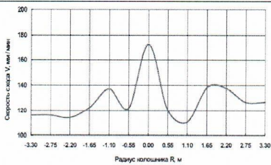
Рис. 5.40. Відеокадр 2 – «Скорість сходу»
